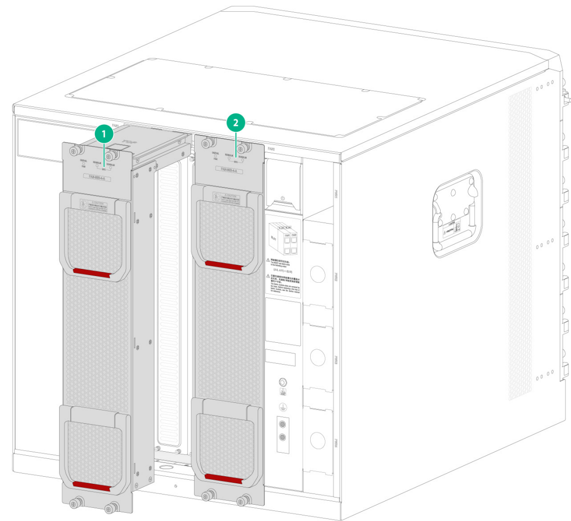
图3-3 风扇框上的网板指示灯与网板槽位对应关系(以 S10600X-06-G 为例)
