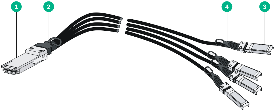
图4-15 QSFP28 to SFP28 DAC 电缆示意图
