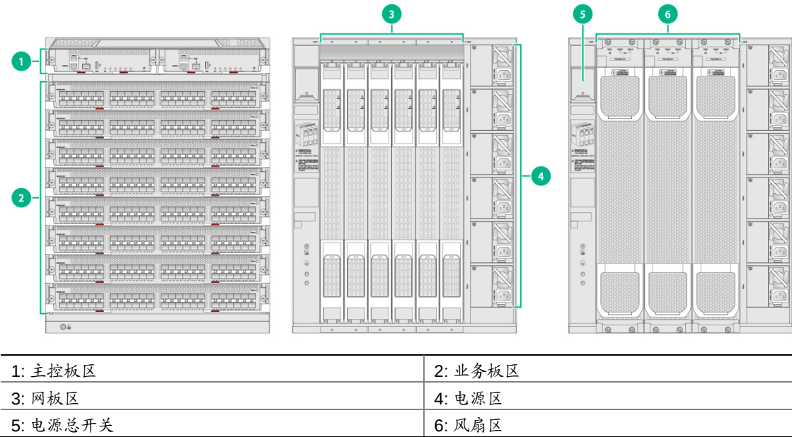
图1-2 S10600X-08-G 系列交换机前、后面板示意图
