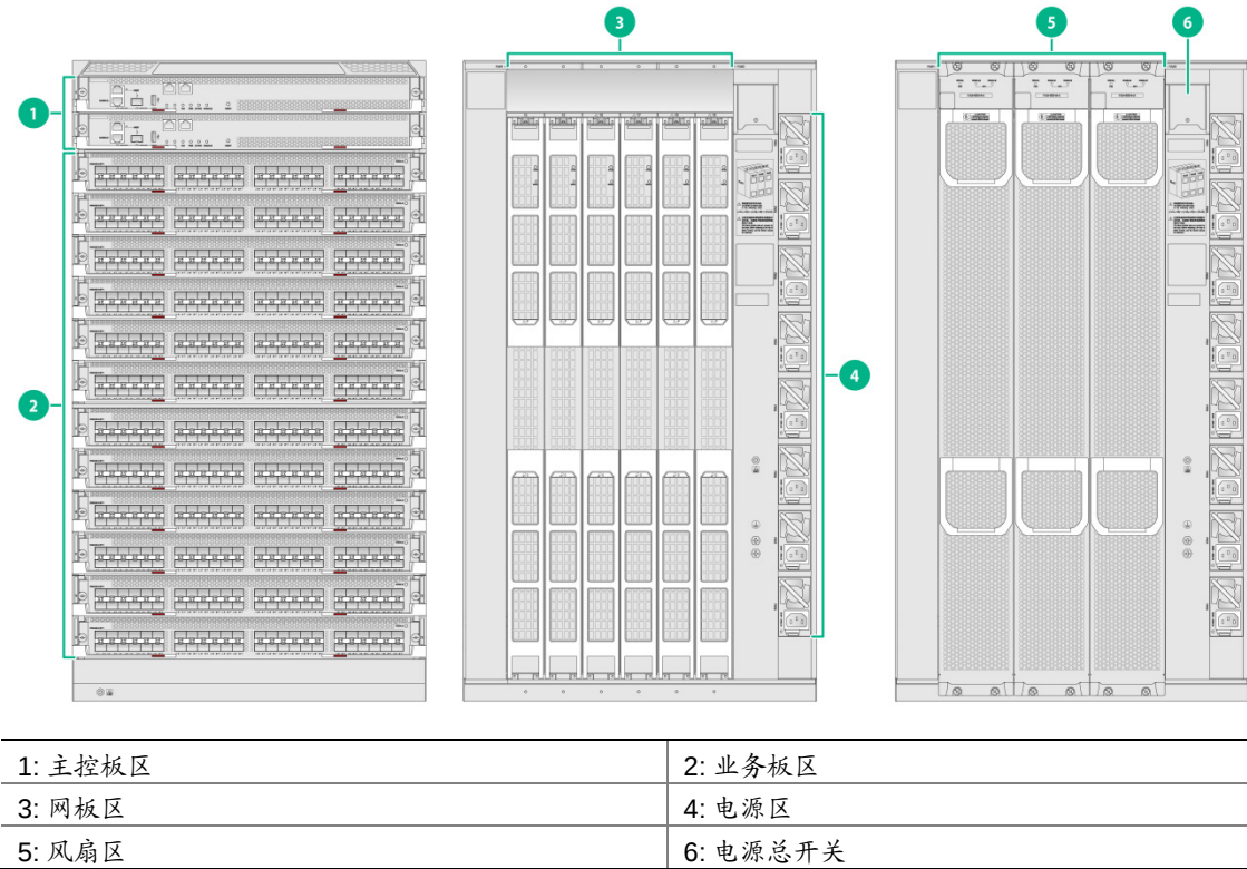
图1-3 S10600X-12-G 系列交换机前、后面板示意图
