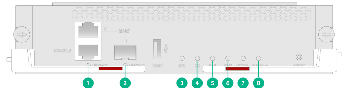
图3-1 主控板 LSEM1SUPA0-Z 指示灯示意图
